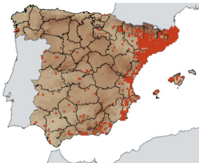
Fig. 4. Distribución de A. donax en la Península Ibérica. Fuente: SANZ ELORZA et al. (2004)
